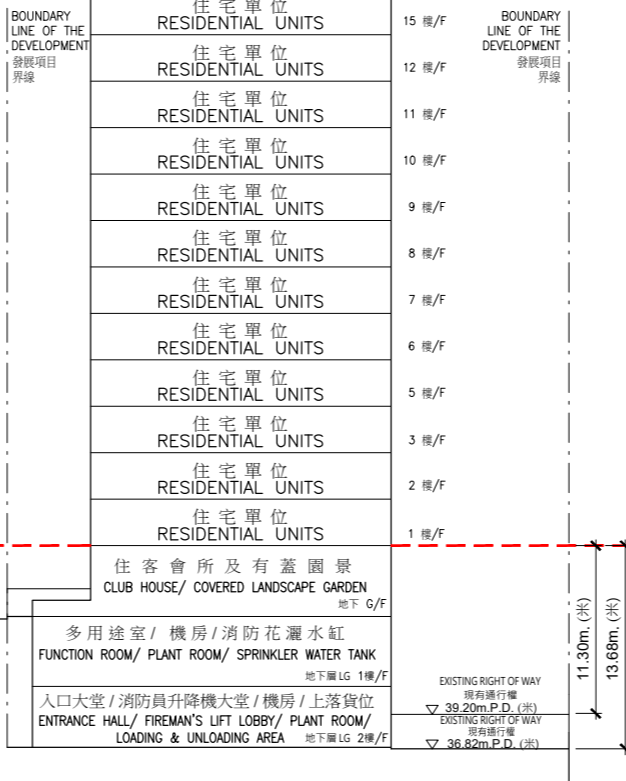
橫截面圖 B
